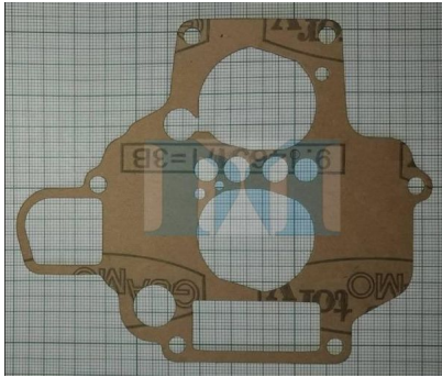
?????????? ?? ??????? ?? ??????????? WEBER 32 DFT
